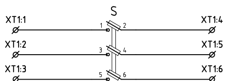
Питание и секционирование цепей блокировки для ШЗВ-60 ... ШЗВ-30
