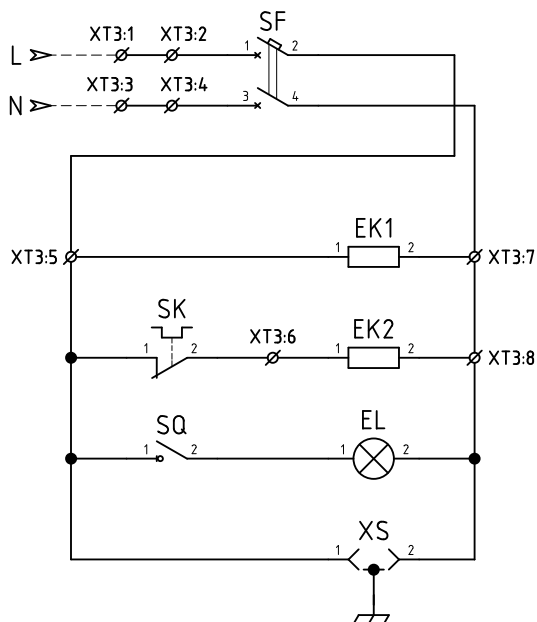
Цепи собственных нужд шкафов ШЗВ-200 ... ШЗВ-30
