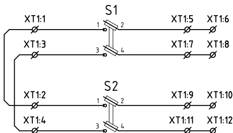
Питание и секционирование цепей блокировки для ШЗВ-200 ... ШЗВ-90
