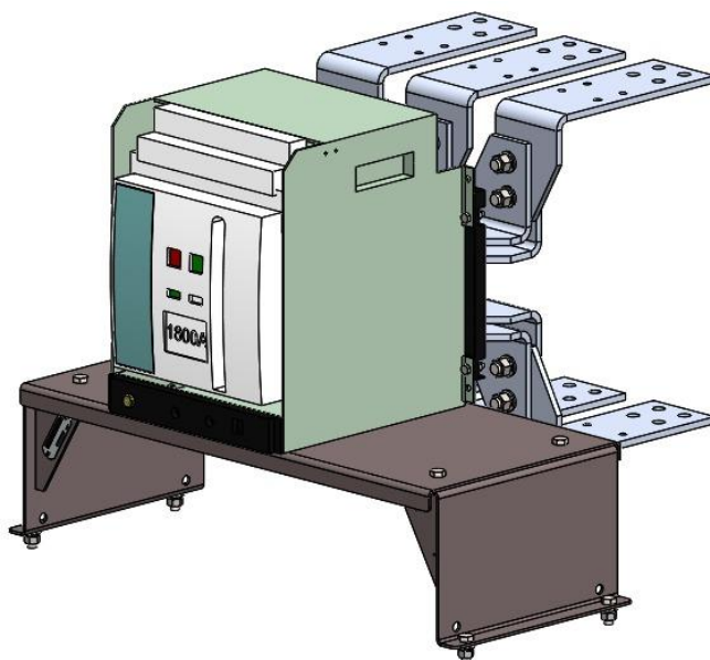
Стационарное, втычное, выкатное исполнение ретрофита НКУ 0,4 кВ
