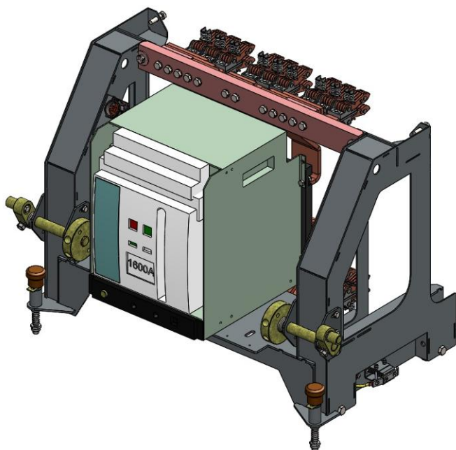
Исполнение ретрофита НКУ 0,4 кВ на тележке аналогичной АВМ
